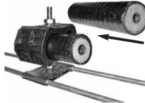
Befestigung-Beispiel für Gitterbahnen Exemple de fixations sur chemins de câble en treillis
